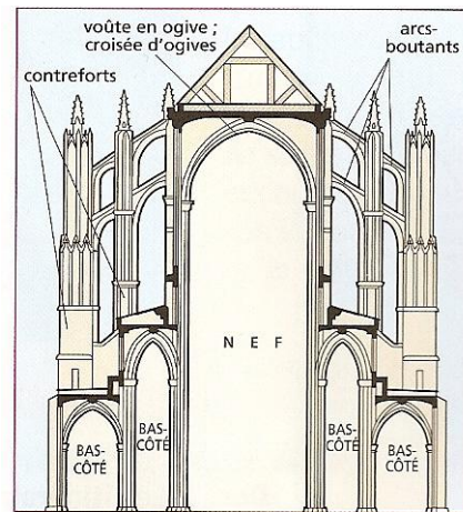
Doc. 6 Coupe d'une église gothique.
