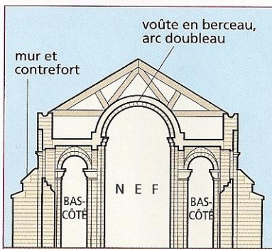
Doc. 5 Coupe d'une église romane.
